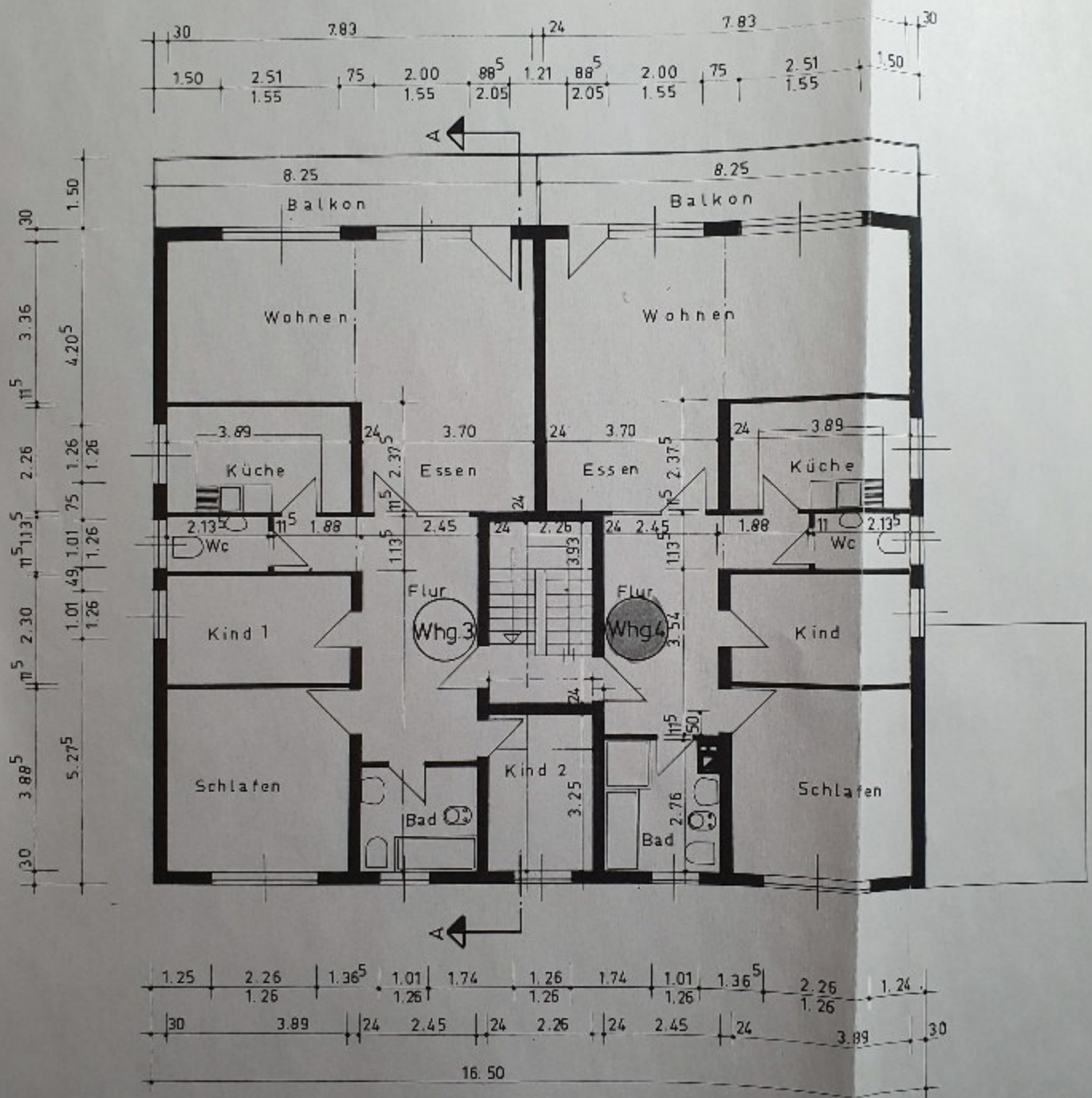
OBERGESCHOSS BESTANDSPLAN
